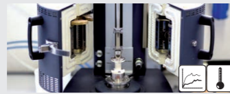
DMA-Messung
